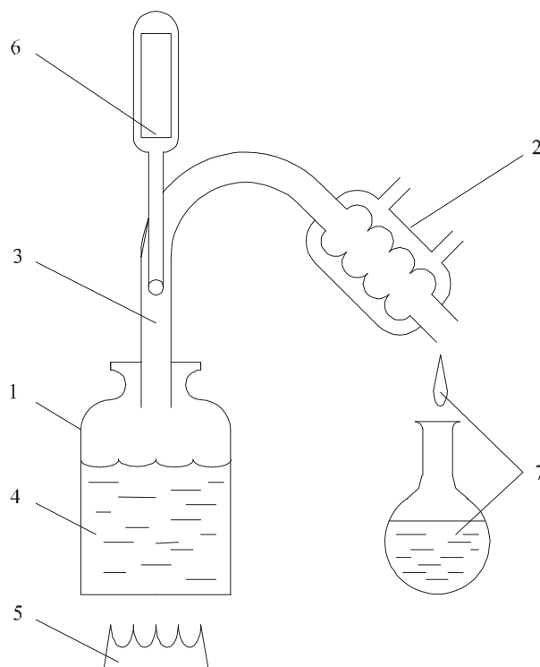
Рис. 2. Схема дистиллятора.
